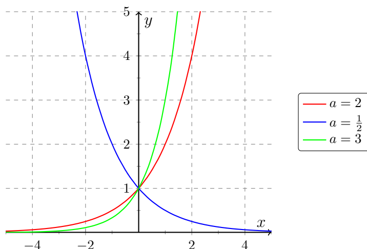
Obrázek 3.14: Exponenciální funkce.
