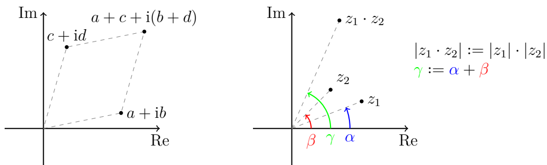
Obrázek 1.6: Geometrická interpretace operace sčítání a násobení komplexních čísel.
