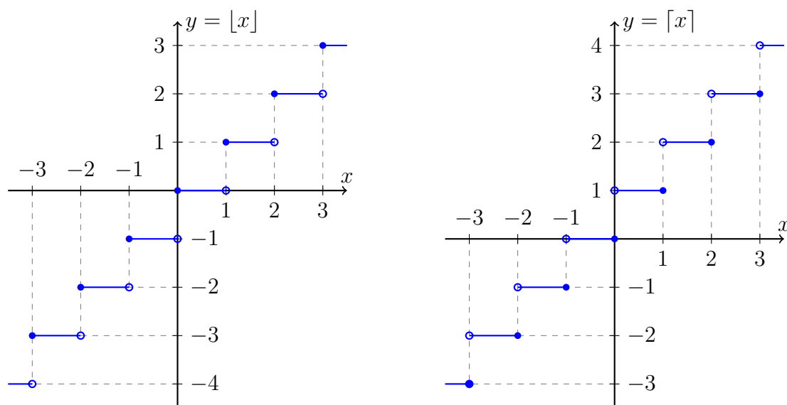
Obrázek 3.2: Grafy dolní (vlevo) a horní (vpravo) celé části.
