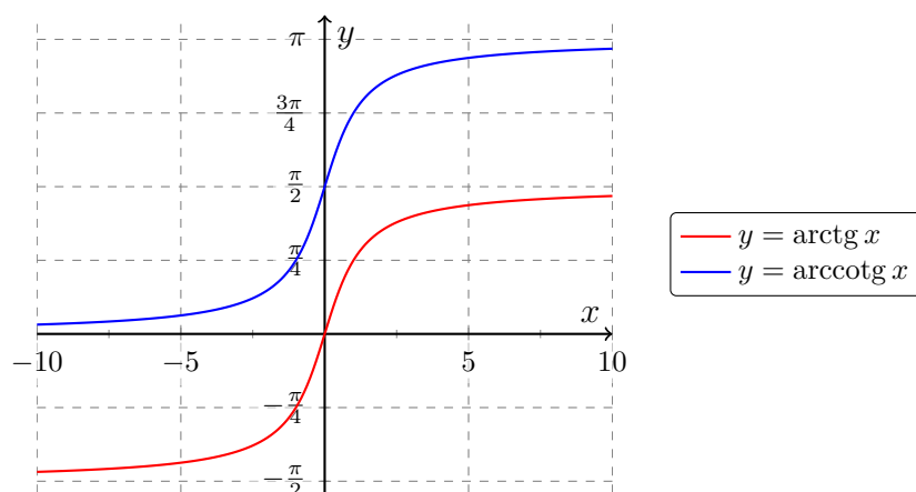
Obrázek 3.13: Grafy funkcí \operatorname{arctg} x a \operatorname{arccotg} x .
