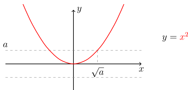
Obrázek 3.5: Ke konstrukci sudé odmocniny čísla a .
