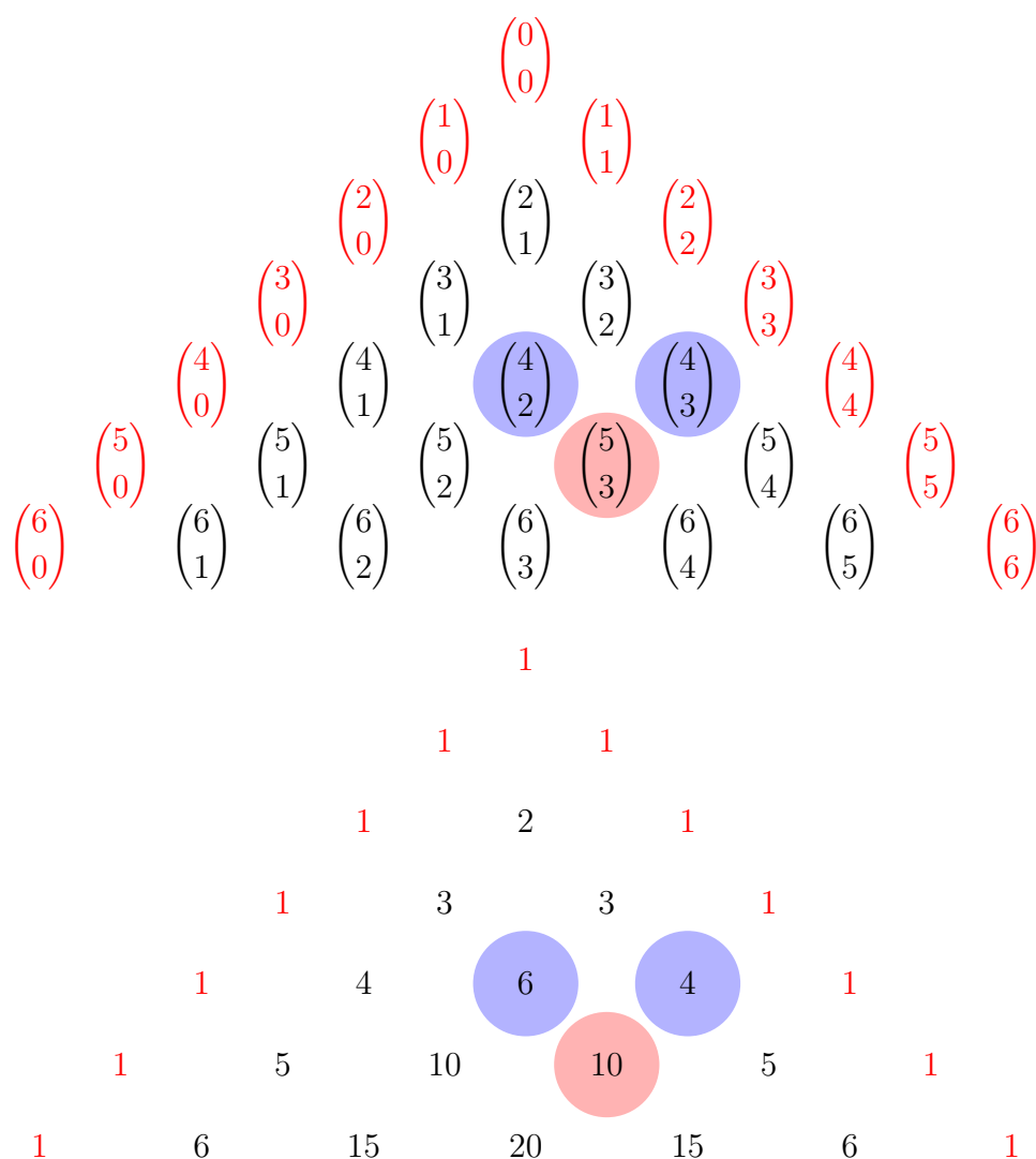
Obrázek 1.8: Pascalův trojúhelník.
