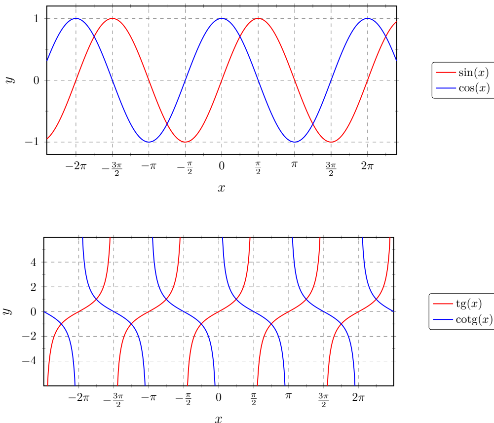
Obrázek 3.11: Trigonometrické funkce \sin , \cos , \operatorname{tg} a \operatorname{cotg} .
