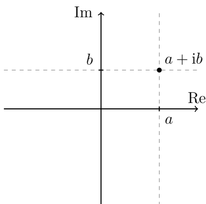
Obrázek 1.5: Komplexní rovina.
